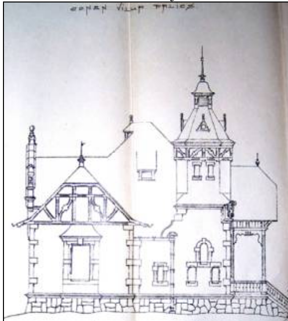
Nacrti paličke vile Konenovih
