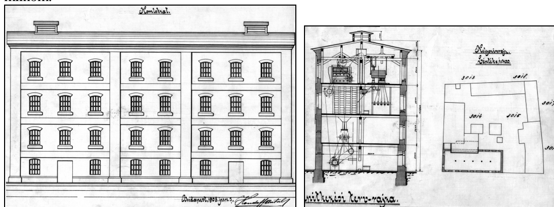
Deo tehničkih planova (1908.g.) mlina Lajče Stantića (kasnije -Margit mlin)
