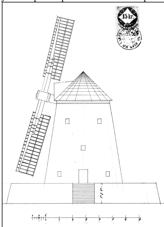
Nacrt vetrenjače u Malom Bajmoku
